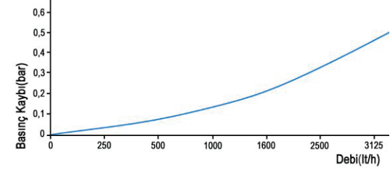
BASINÇ KAYBI GRAFİĞİ(PRESSURE LOSS GRAPH)
