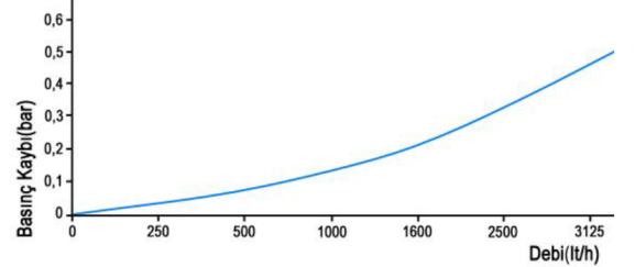
BASINÇ KAYBI GRAFİĞİ(PRESSURE LOSS GRAPH)
